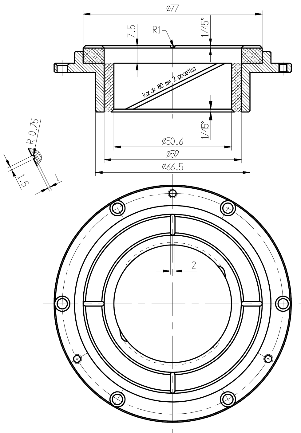
LEŽAJ RADIJALNO-AKSIJALNI DESNI (ZADNJI) LTCT 100123
